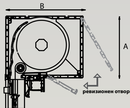
Кутия за вграждане с изолацията от вътрешната и от външна страна
