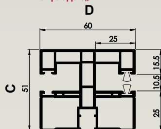
ПВЦ водач „Н“
