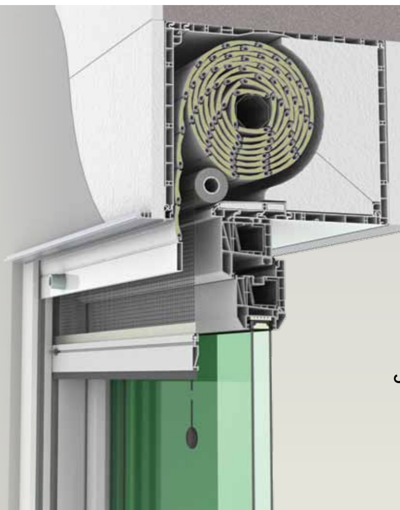
Кутия за вграждане с изолацията от вътрешната и от външна страна
